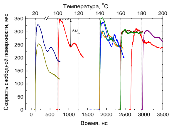
Рисунок 1 – Профили скорости свободной поверхности образцов поликарбоната
