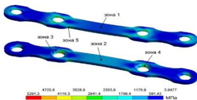
Рис. 1. Эквивалентные напряжения в пластинах из УМЗ титана при расчетной нагрузке 1200 Н
