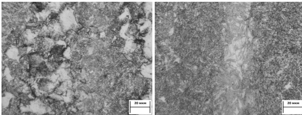
Рис. 3. Микроструктура стали 30X3МФА после охлаждения от температуры 900 °С со скоростью 0,1 °С/с (а) и 0,3 °С/с (б)
