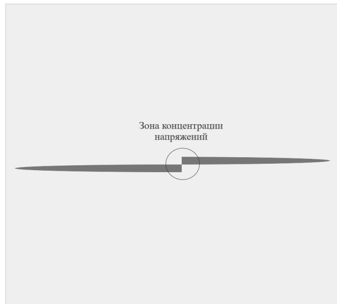
Рисунок 1. Разлом со ступенчатым усложнением.
