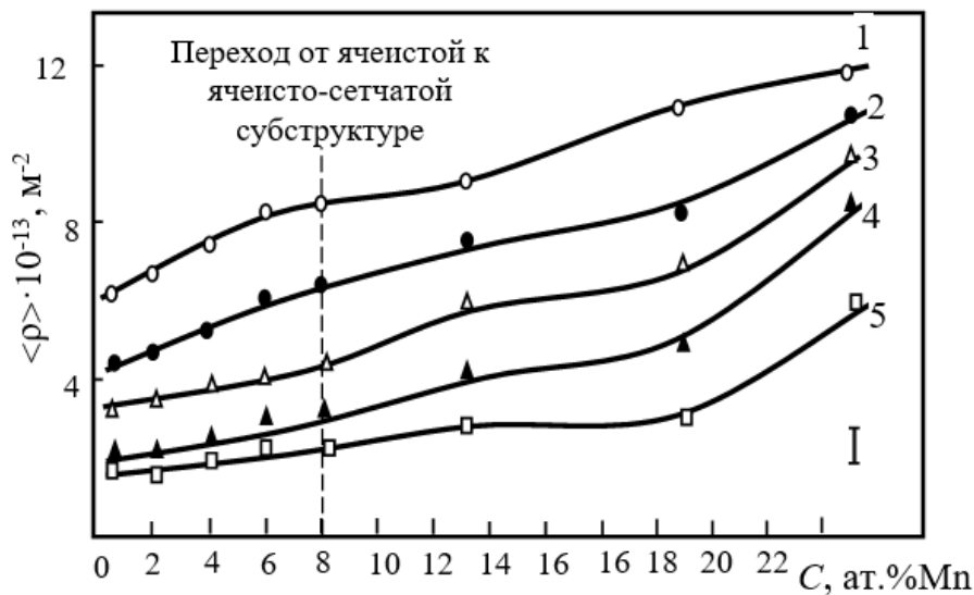
Рисунок 2. Зависимости средней скалярной плотности дислокаций \langle \rho \rangle от концентрации легирующего элемента C марганца при разных размерах зерен и степени деформации \epsilon_{ист} = 0.05 : 1 – d = 20 \text{ мкм} ; 2 – d = 40 \text{ мкм} ; 3 – d = 60 \text{ мкм} ; 4 – d = 120 \text{ мкм} ; 5 – d = 240 \text{ мкм} . Пунктирной линией показан переход от ячеистой к ячеисто-сетчатой субструктуре. T_{деф} = 293 \text{ K}
