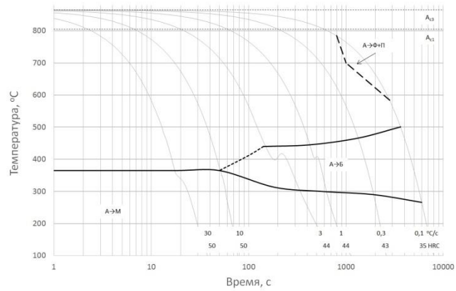
Рис. 2. Термокинетическая диаграмма превращения переохлажденного аустенита в стали 25X2ГCMA (а) и 30X3МФА (б)
