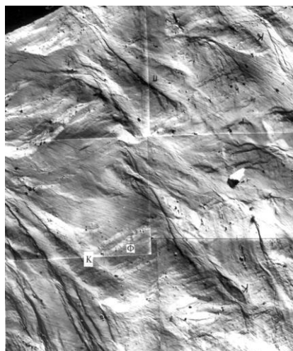
Рисунок 1. Деформационные складки в стали 34XN3MFA
