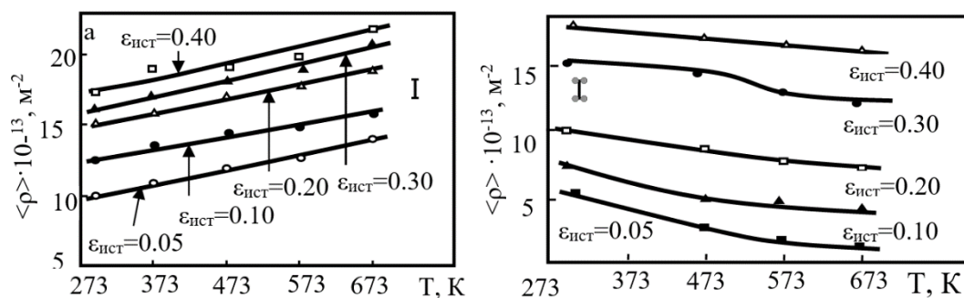
Рисунок 3. Зависимости средней скалярной плотности дислокаций ( \langle \rho \rangle ) от температуры испытания (Т): а – сплав Cu+14ат.%Al, б – сплав Cu-19ат.% Mn при разных степенях деформации ( \epsilon ). Размер зерна d = 40 мкм
