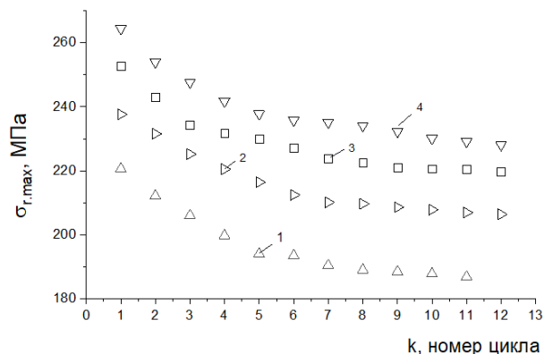
Рисунок 1. Зависимость реактивных напряжений сплава Ti_{50}Ni_{40}Cu_{10} от номера цикла при первоначальной нагрузке: 1 – 27 МПа; 2 – 40 МПа; 3 – 53 МПа; 4 – 66 МПа
